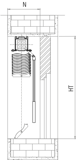
Argano diretto - Crank motor with direct joint for handle
