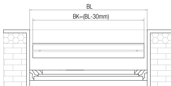
Sezione orizzontale guida a cavo horizontal section with cable guides
